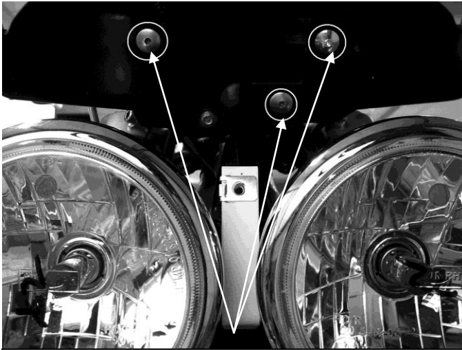
Position des vis de fixation du tableau de bord
